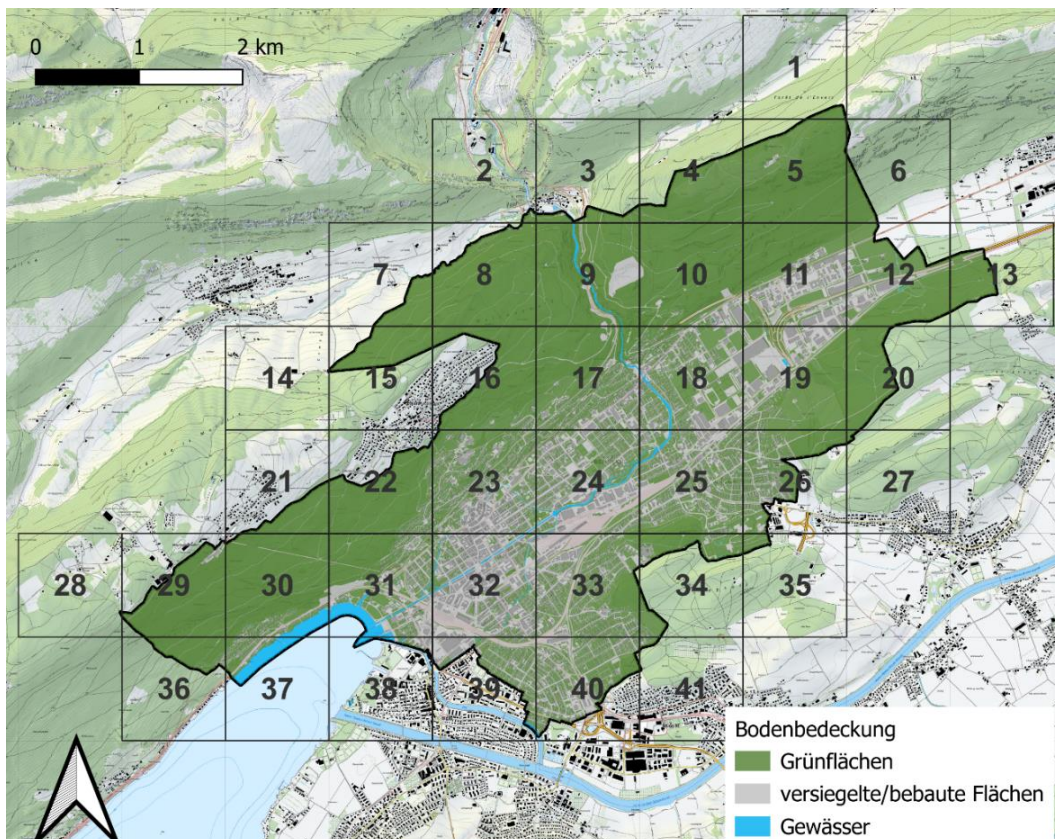
Abbildung 1: Bodenbedeckungskarte der Stadt Biel mit eingeteilten Kilometerquadraten (Hintergrund: MOPUBE - Amtliche Vermessung, Bodenbedeckungskarte der Stadt Biel, Swisstopo, abgeändert durch Prona AG, 21.10.2024)
